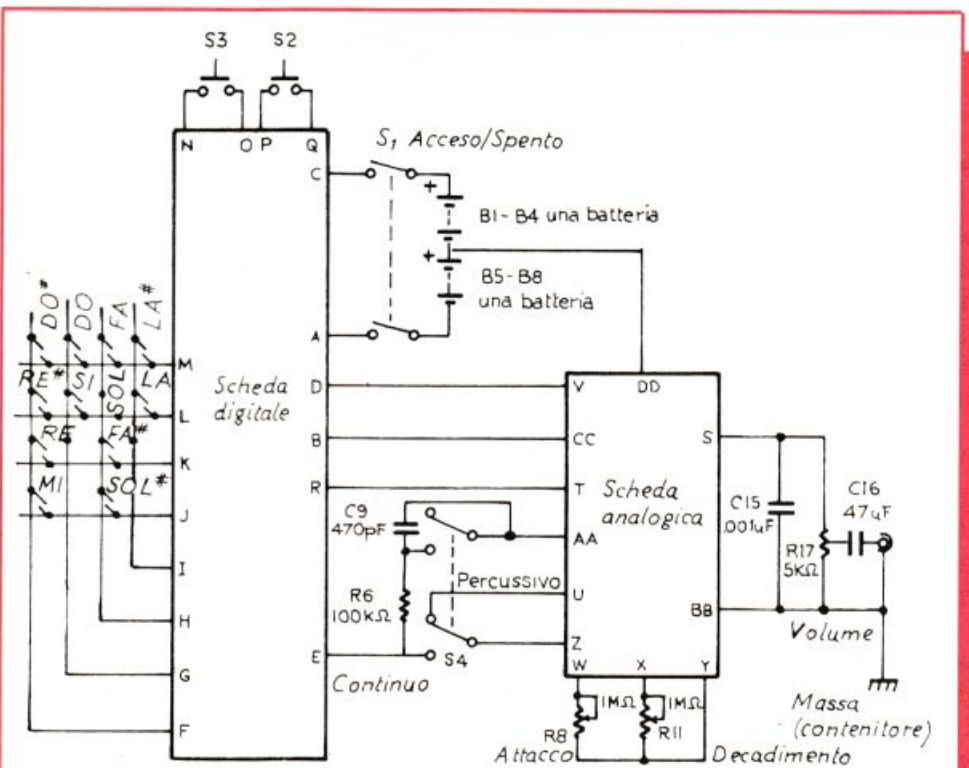
Figura 2. Le varie note che vengono generate dal clarinetto digitale sono create dalla circuiteria alloggiata dalla scheda digitale. Gli altri comandi fanno capo alla scheda analogica.
